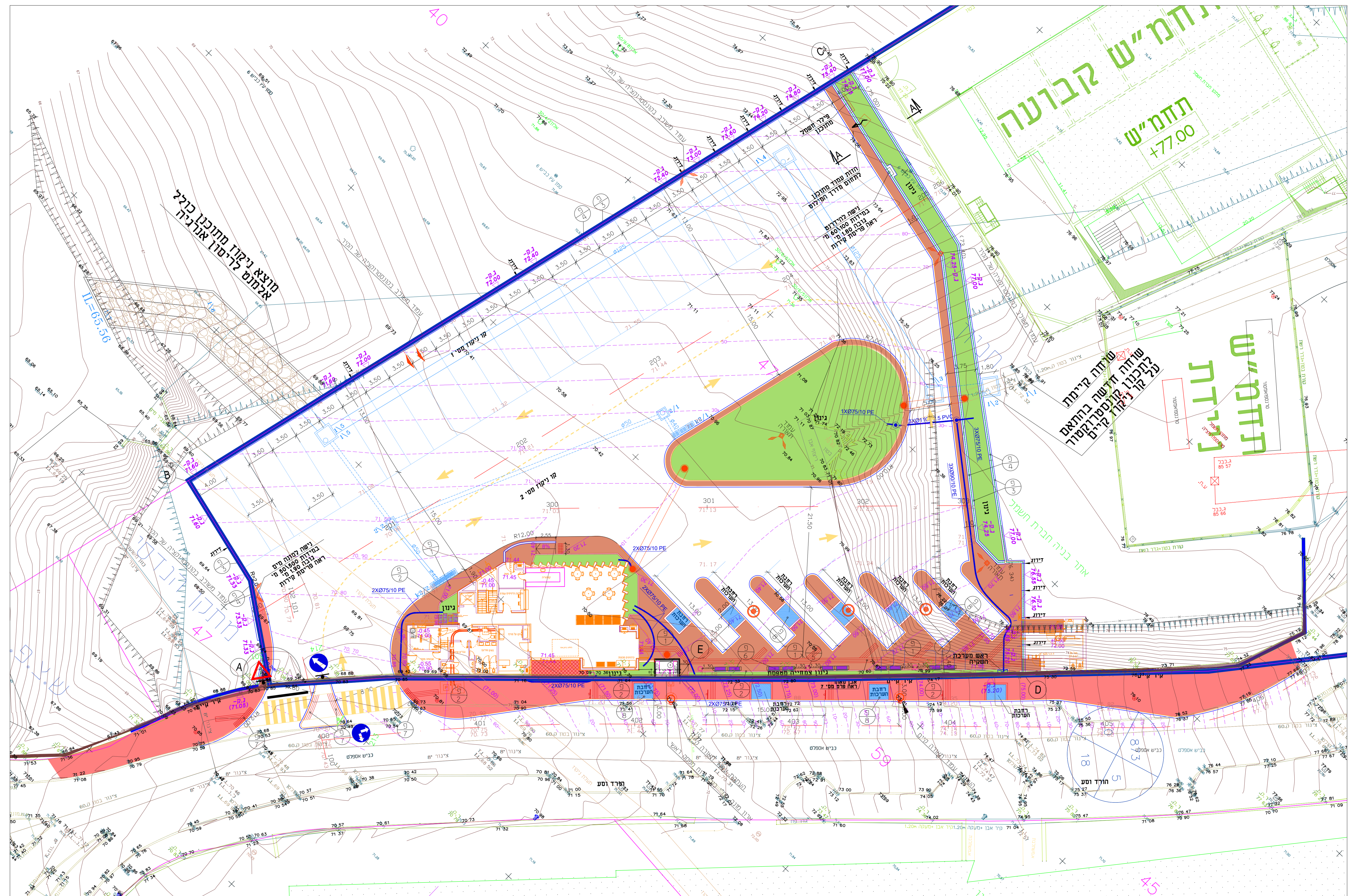
תכנית פיתוח קני"מ: 1:200
